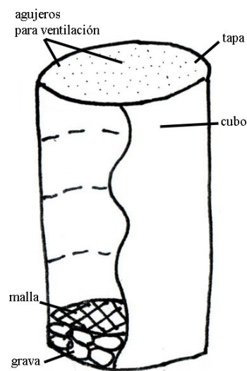
Vermicompostera con un cubo
